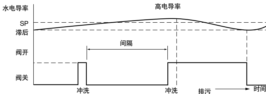
图7 带冲洗时间设置的输出 (冲洗时间>0秒)
