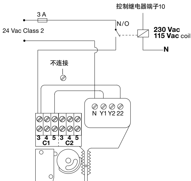
图19 UL24V交流BCV30 阀门接线图
