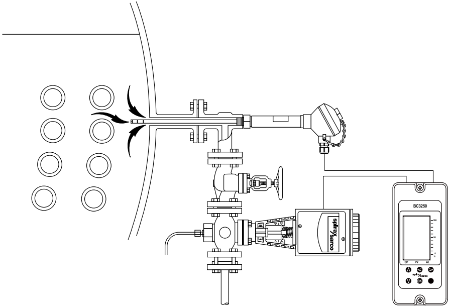
图11 BCS3系统-带一体排放TDS控制及锅炉侧连续监测
