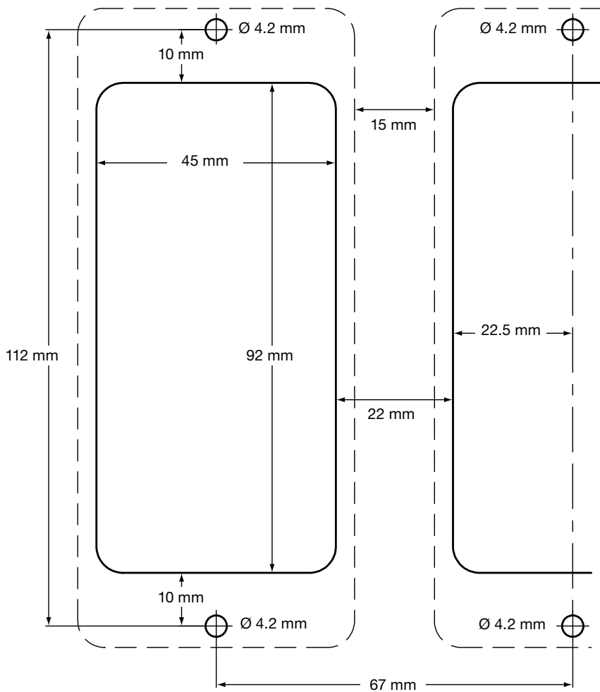
图15 底板/面板-剪裁图
