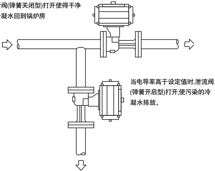
图14 使用两个阀的CCD系统布置
