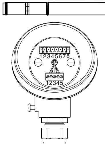
图27旧型CP32 (不带脉冲电路) 选择: PULSED
