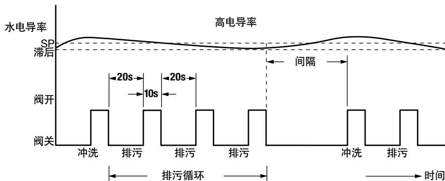
图8 带冲洗时间设置的脉冲输出 (冲洗时间>0秒)
