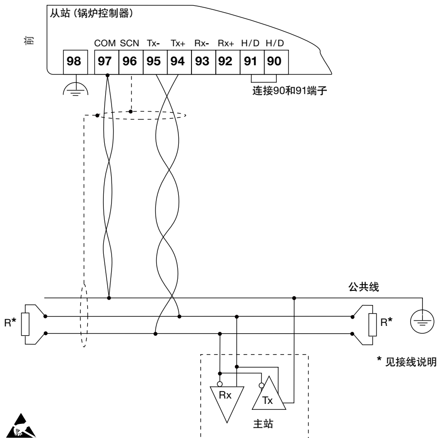
图24 RS485/Modbus半双工回路 (顶视图)
