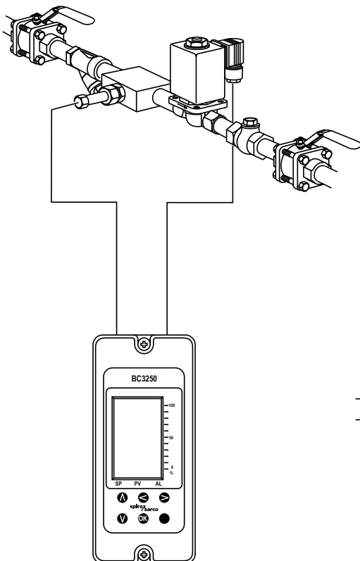
图9 BCS1 系统-小锅炉
