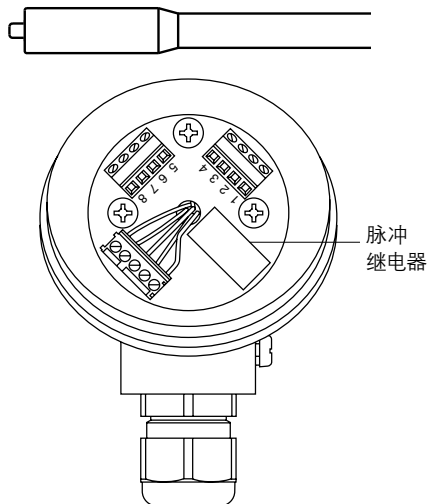
图27新型CP32 (带脉冲电路) 选择: CONSTANT
