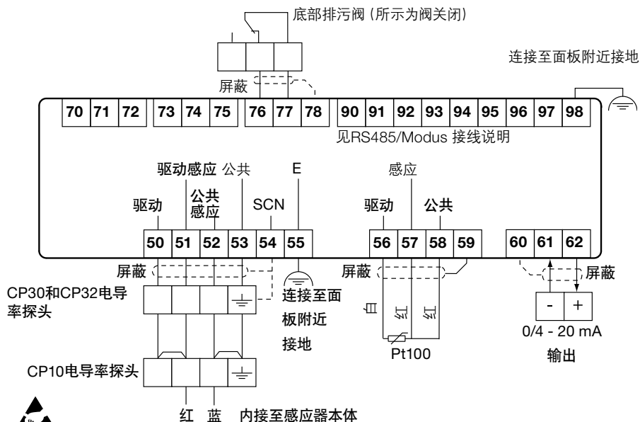
图21 信号回路 (顶视图)
