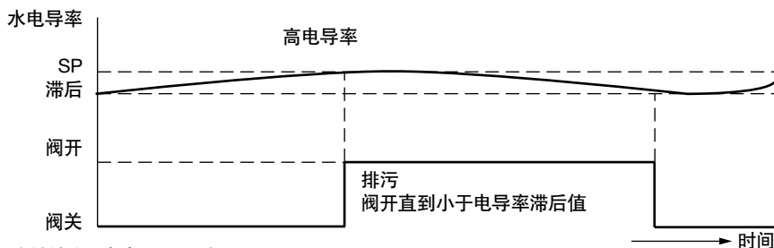
图6 连续输出 (冲洗时间=0秒)
