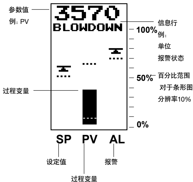
图2 图形定义-条形图模式
