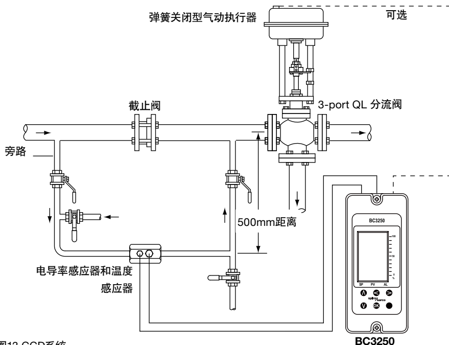
图13 CCD系统
