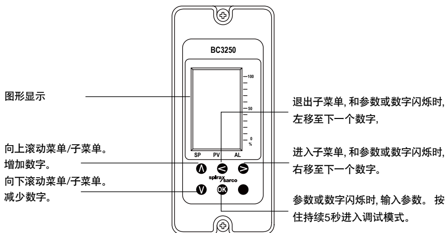
图1, 前端面板及定义
