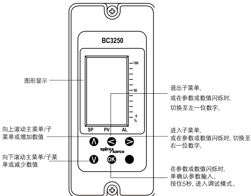
图25 前端面板按钮及定义
