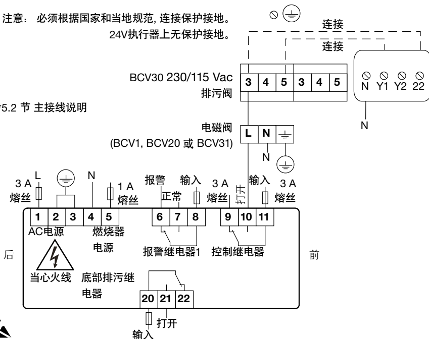
图18 主回路（底视图）继电器在失电位置
