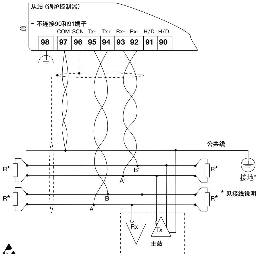
图23 RS485/Modbus 全双工回路 (上视图)
