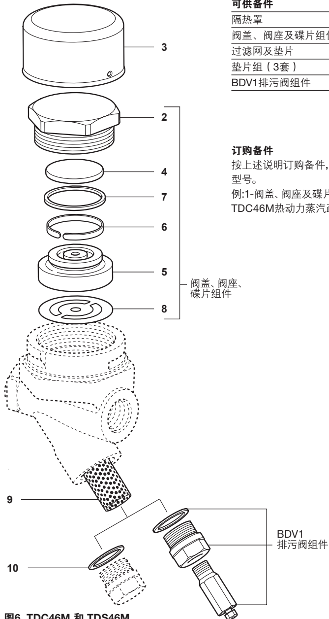
图6 TDC46M 和 TDS46M
