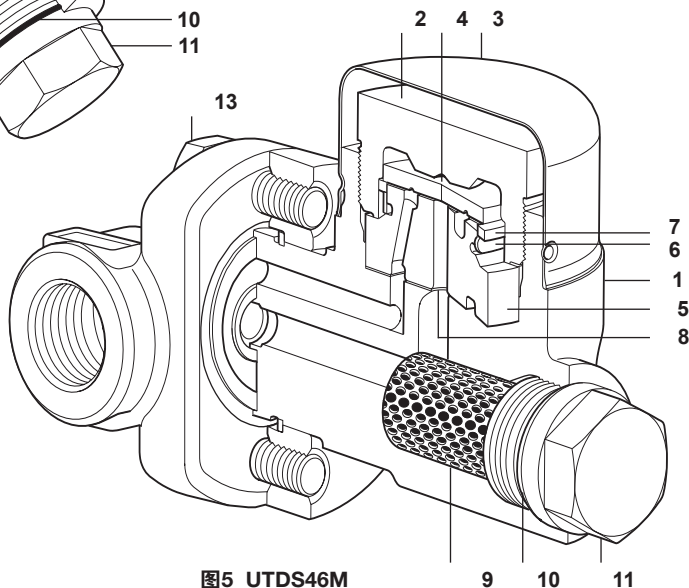
图5 UTDS46M
